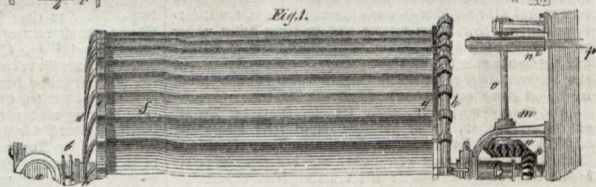
Crabdoe's Condensator für Locomotiven.
