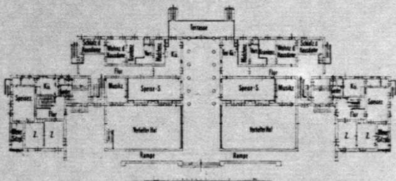
Mittleres Wohnhaus. Erdgeschoß.
