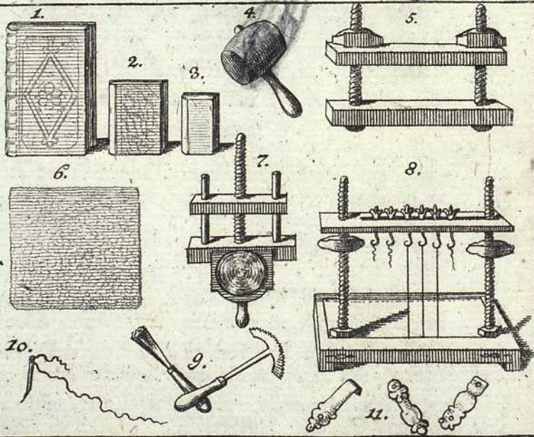
1. Folio Band. 2. Quart Band. 3. Octav Band. 4. Hammer. 5. Presse. 6. Papendeckel. 7. Hobel. 8. Hestlade. 9. Zie- rathen Stempel. 10. Nadel und Faden. 11. Klausuren. N. Gabelndel. No 44. Pemsel sc.
