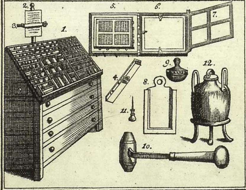
1. Der Schriffkasten. 2. Tenackel. 3. der Zeilenweiser. 4. Winkelhacken. 5. Form. 6. Decktel. 7. Rahm. 8. Schiff. 9. Ballen. 10. Bengel. 11. Ahle. 12. Kessel.
